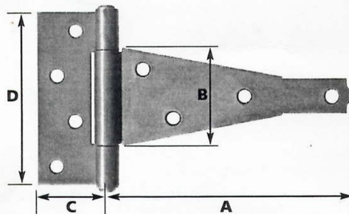
TEE HINGE
